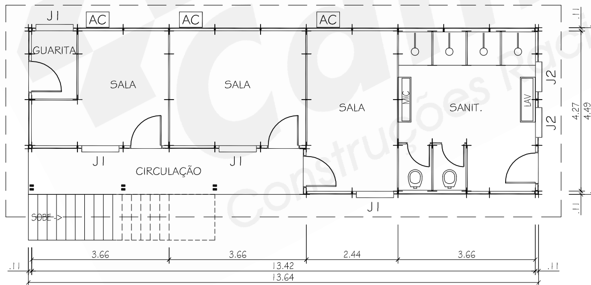
PLANTA - PAVIMENTO INFERIOR
