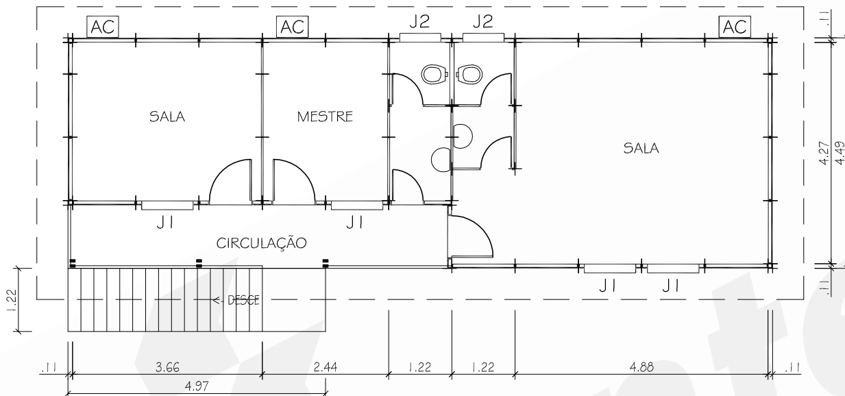
PLANTA - PAVIMENTO SUPERIOR
