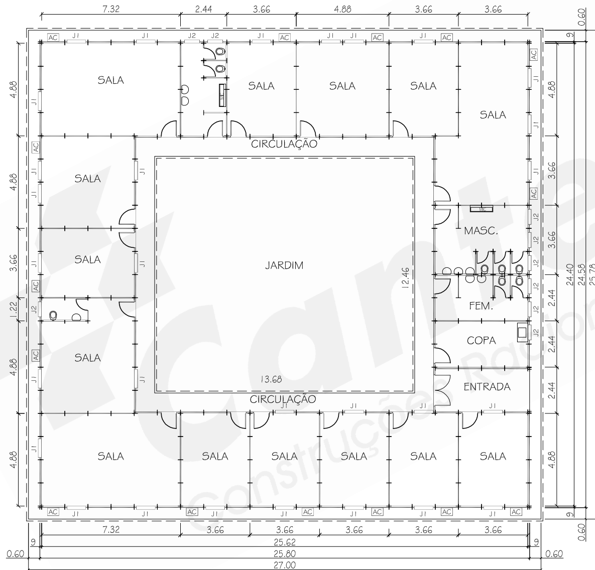
PLANTA
